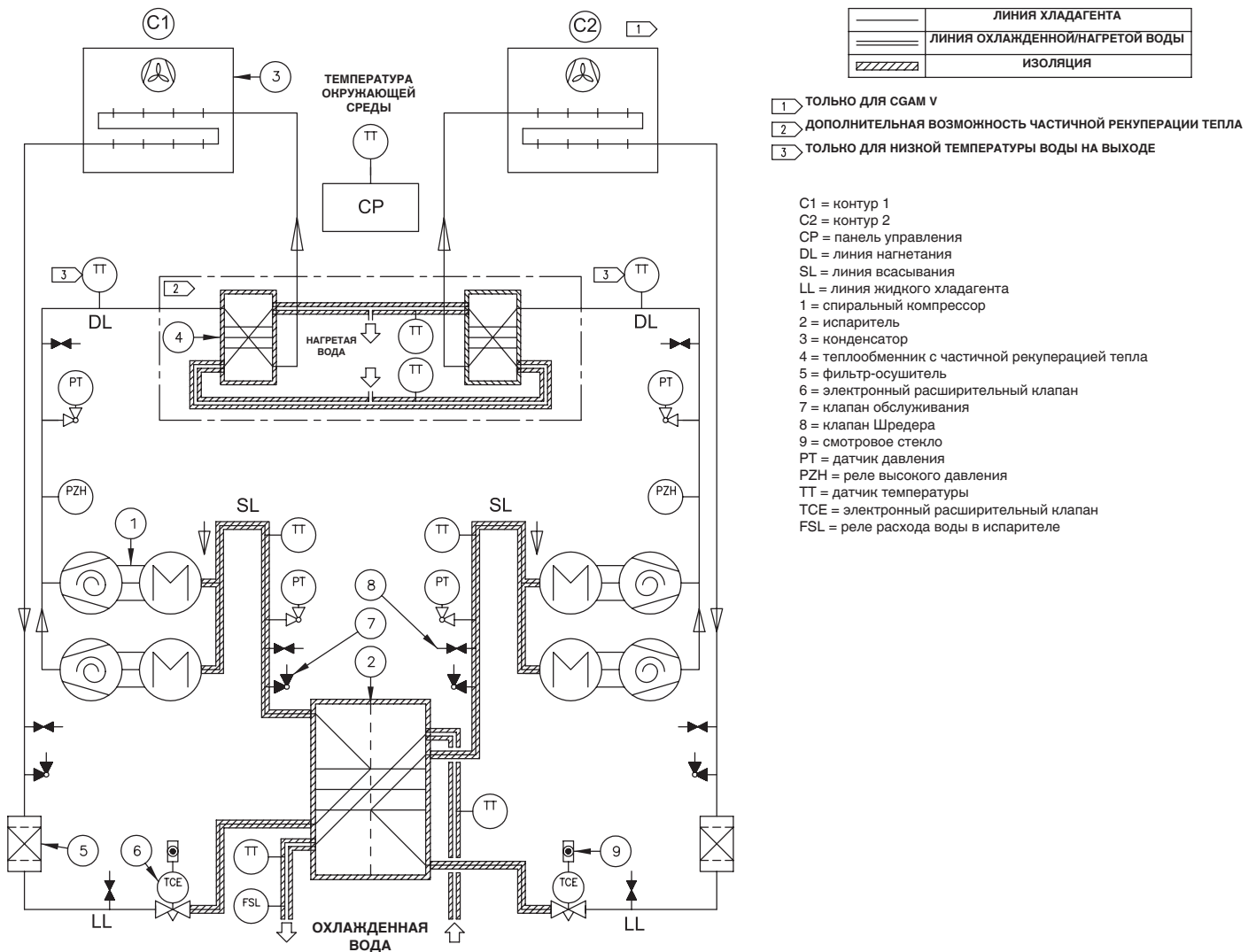
Рисунок 28 - Контур хладагента CGAM - Конфигурации теплообменника S и V
